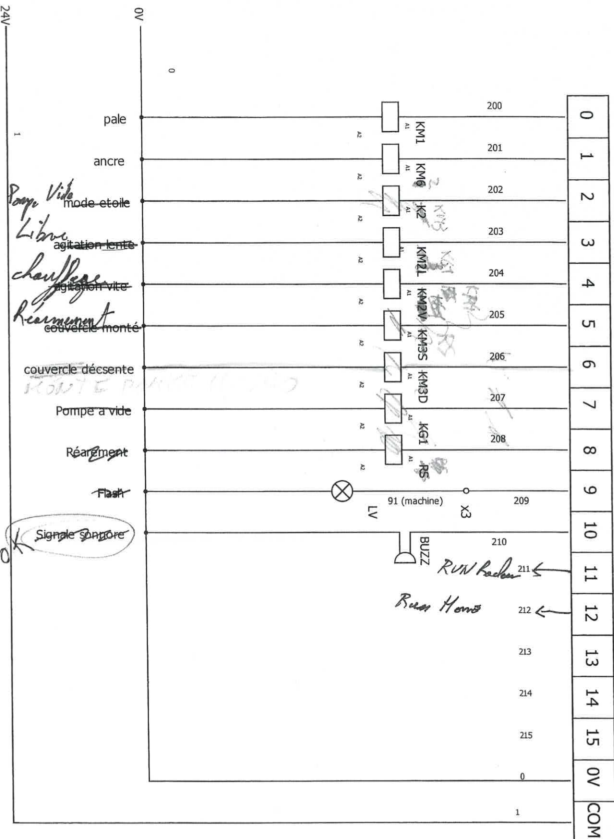
Schéma sortie automate 1/2
